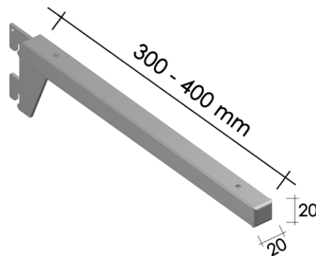
Braço Reto 20x20
