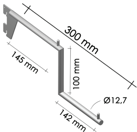
Braço Dois Níveis Maciço Ø12,7
