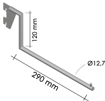
Braço Descendente Maciço Ø12,7
