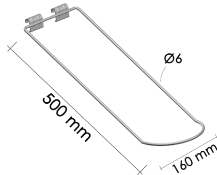
Suporte Duas Bolas para Régua
