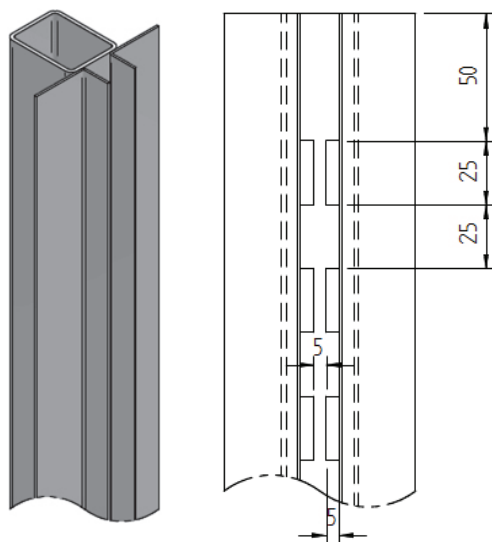
Com capa Estampada 1 lado
