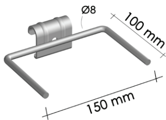
Suporte Calçados "U" para Régua
