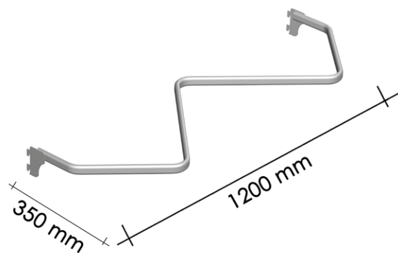
Expositor "W" 30x16
