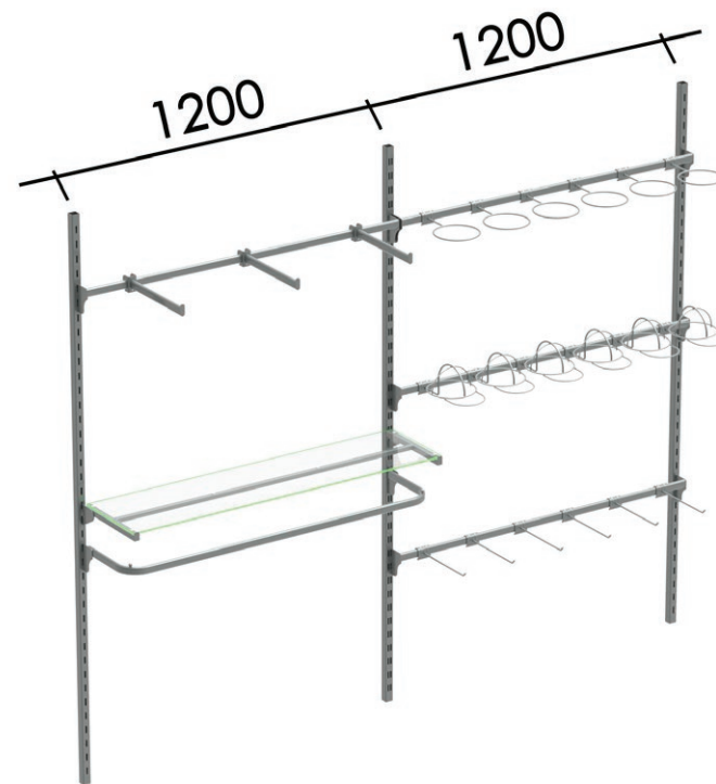
Módulo 1200mm - Cremalheira 30x30 sem capa
