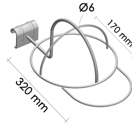
Suporte Boné p/ Régua
